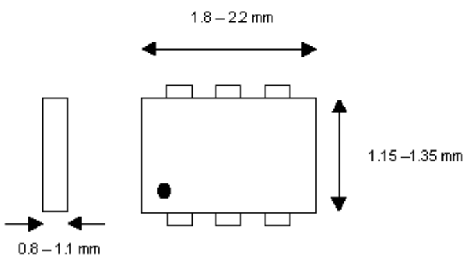
SOT-363
